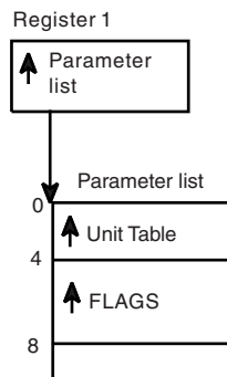
Figure A-1. Input Parameter List
